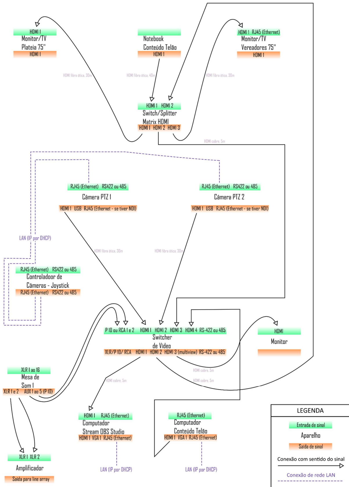
Diagrama de Conexões de Entrada/Saída dos Sistemas de Câmeras, Telas e Áudio
